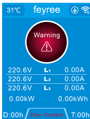
Виявлено надструм
