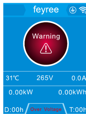
Виявлено перенапругу
